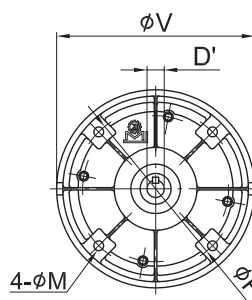
入力孔 INPUT BORE
