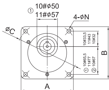
SVD-A法蘭面
